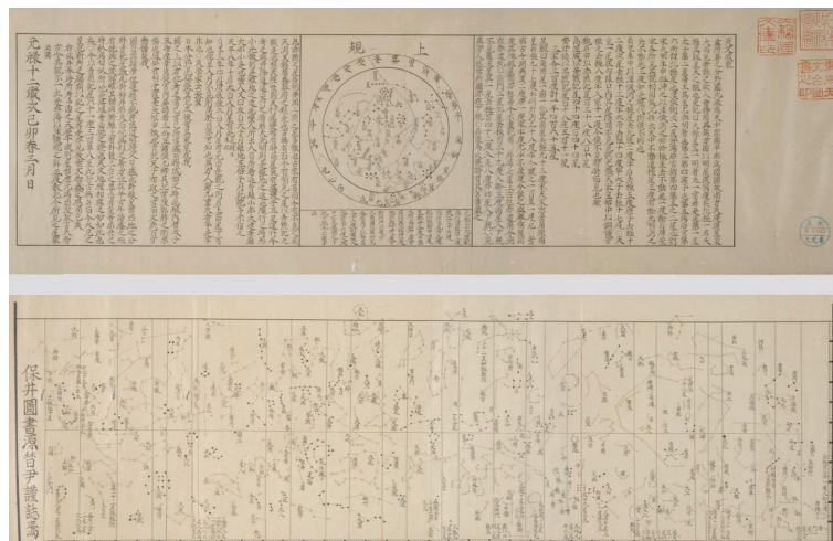
図 18: 保井昔尹・渋川春海『天文成象』(1699 年)の部分. 渋川春海自身の観測に基づいて, 中国星図に 308 星追加した. 画像は国立天文台より取得. Fig. 18: Celestial map by Hisatada Yasui & Harumi Shibukawa (1699).
