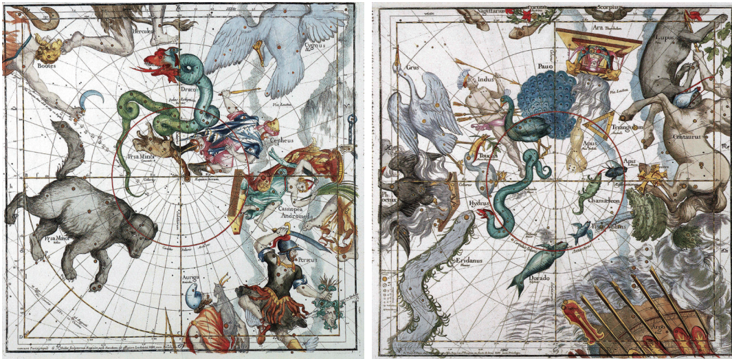
図 3: イグナス・パルディによる天球図 (1674 年). 北天図 51.2 cm×78.6 cm, 南天図 51.7 cm×78.5 cm, 正像星図であり, 中心は天の北極と南極. 黄道座標も点線で表示されている. 千葉市立郷土博物館蔵. 画像は『星座の文化史』(千葉市立郷土博物館蔵, 1995) より.
