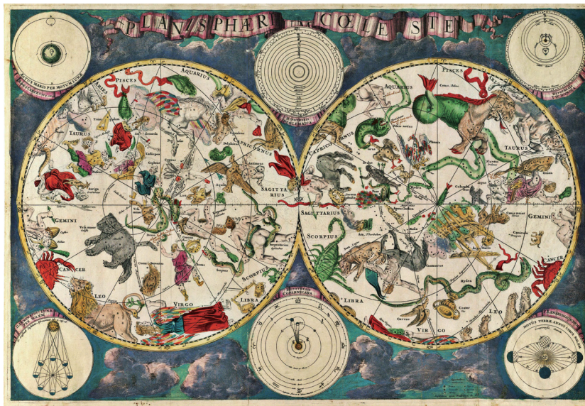
図 2: デ・ウィットによる天球図 (1670 年)。反転星図であり、北天図・南天図とも中心は黄極。司馬江漢が天球図のもとにしたと考えられるもの。画像は Wikipedia より取得。
