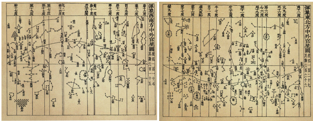
図 13: 蘇頌『新儀象法要』(1094 年)にある方図. 徐剛, 王燕平著『星空帝国』(楓樹林出版, 2019)より. Fig. 13: Celestial map by Soshou (1094).
