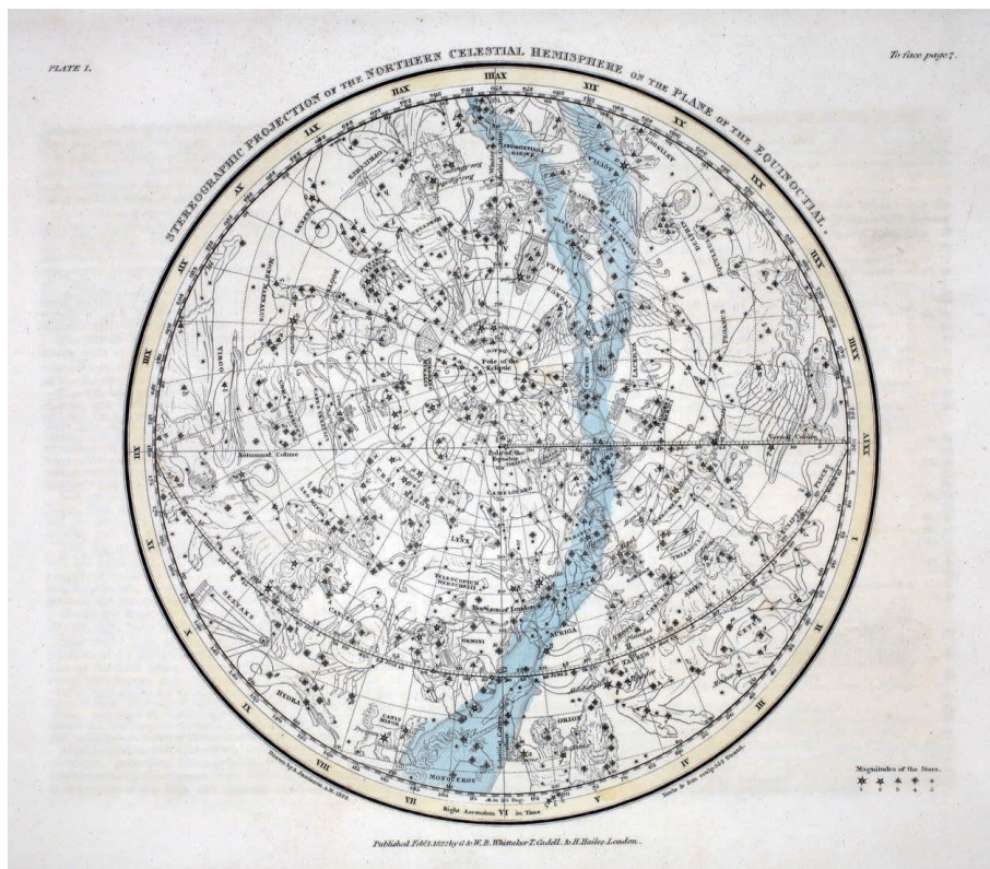
図 11: ジェイミソンによる天球図 (1822 年). 正像であり, 赤道座標が使われている. 黄道座標も点線で入っている. 星は 5 等星まで書き込まれている. 星座図が入ったものとしては, ほぼ最終形. インターネットより取得. Fig. 11: Celestial map by Alexander Jamieson (1822).
