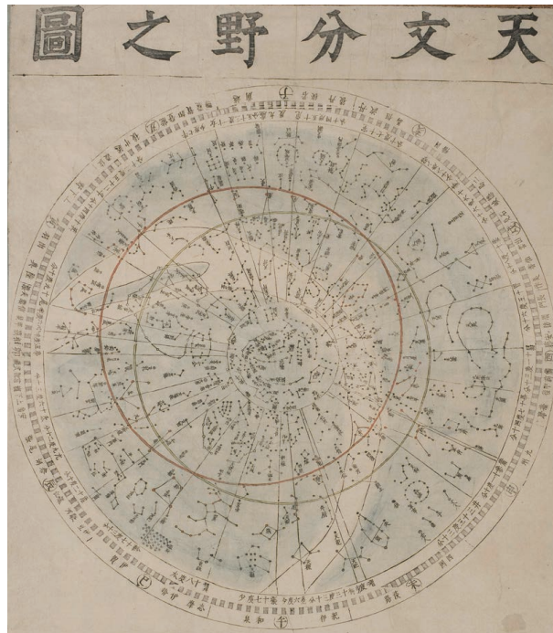
図 17: 渋川春海『天文分野之図』(1677 年)の部分. 二十八宿の星は赤く彩色されている. 画像は国立天文台より取得. Fig. 17: Celestial map by Harumi Shibukawa (1677).
