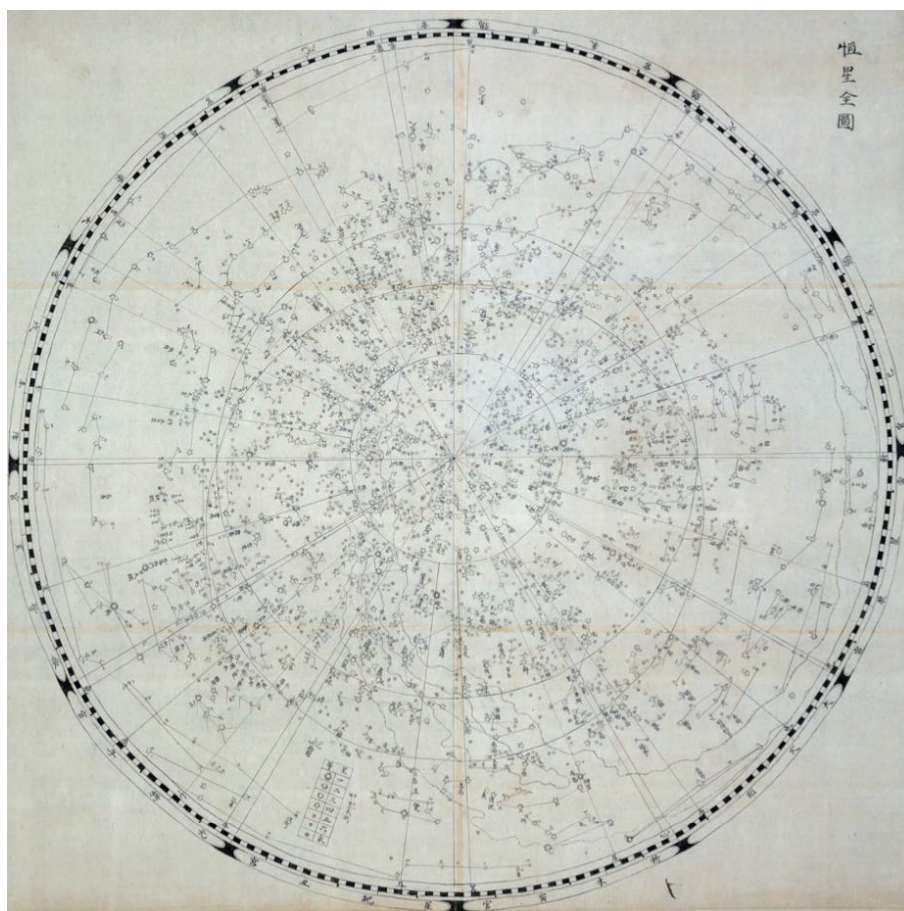
図 19: 伊能忠誨『恒星全圖』(1825 年). 6 等星まで区別されて描かれている. 伊能忠敬記念館所蔵. 画像はインターネットより取得.
