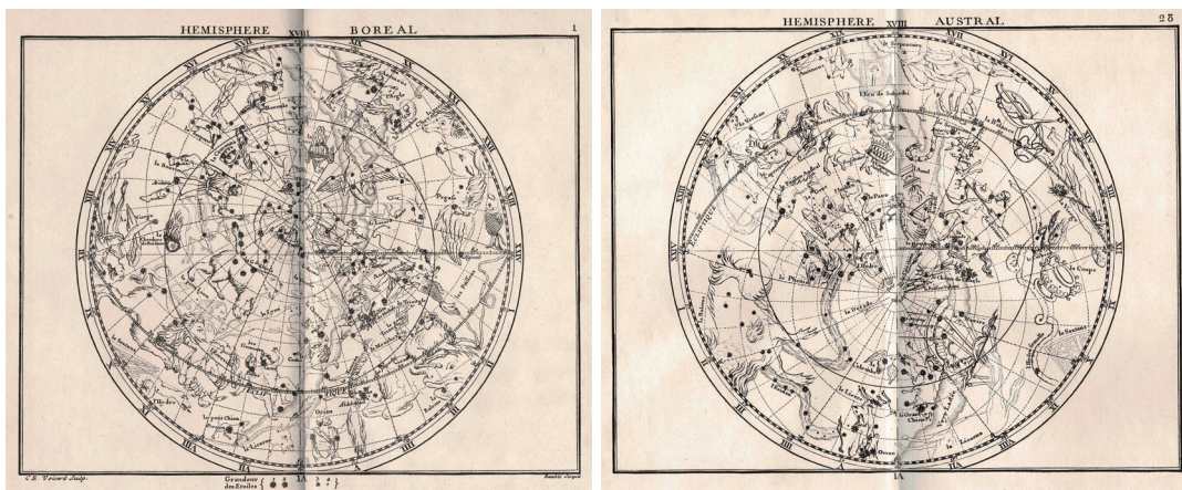
図 8: フラムスティードによる天球図 (1729 年). 正像であり, 赤道座標, 黄道座標も点線で記入されている. 『フラムスチード天球圖譜』(恒星社, 1943) をスキャンしたもの.
