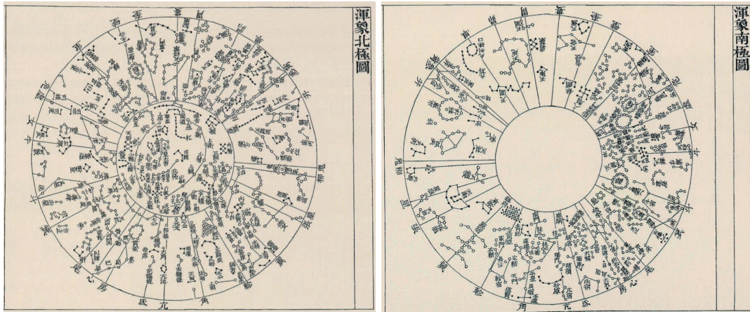
図 12: 蘇頌『新儀象法要』(1094 年)にある北天図と南天図. 徐剛, 王燕平著『星空帝国』(楓樹林出版, 2019)より. Fig. 12: Celestial map by Soshou (1094).
