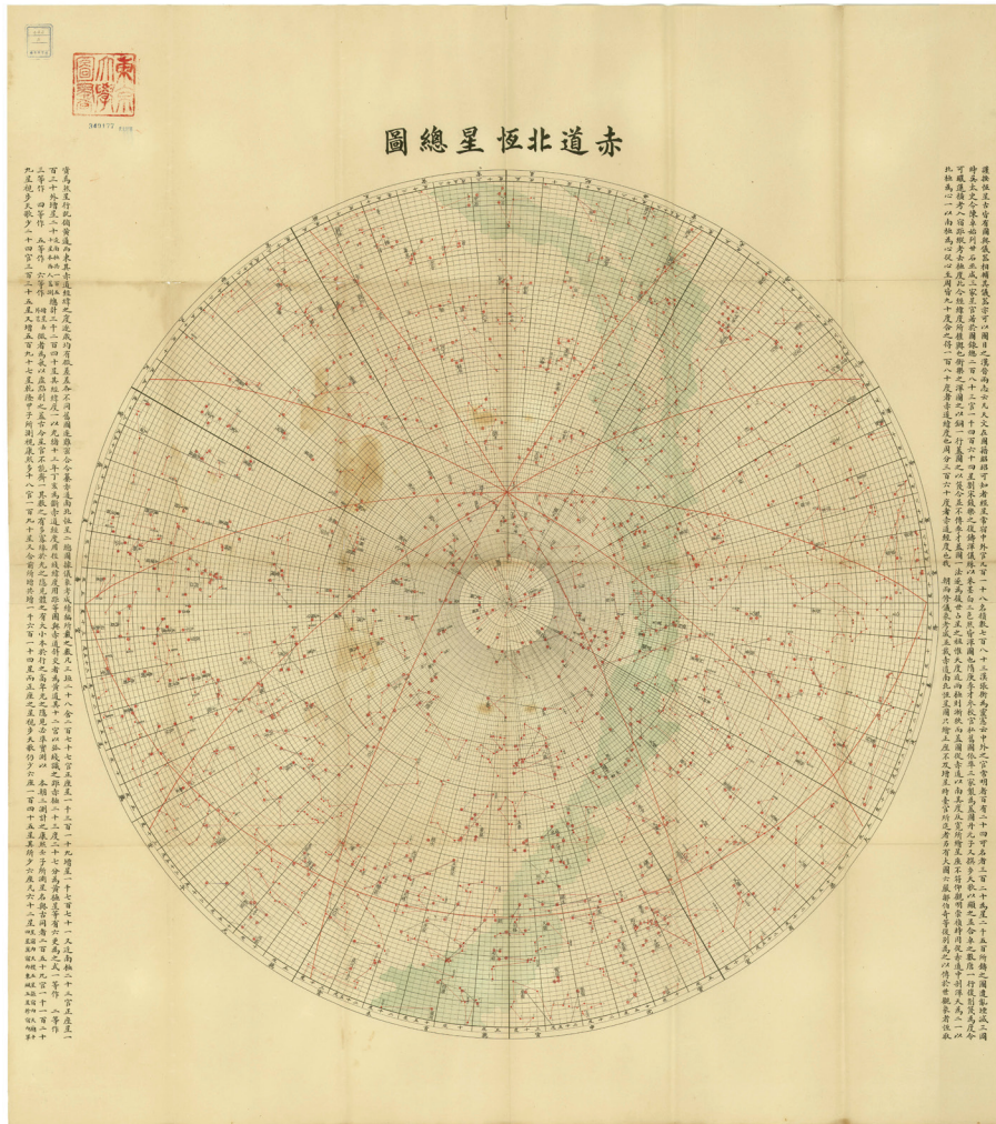
図 16: 『儀象考成続編』の「赤道北恒星総図」(1845年). 赤道座標が細かく記載されていて, なおかつ黄道座標も記入されている. 星は4段階の明るさで描き分けられている. 国立天文台のページから. Fig. 16: Celestial map of 儀象考成続編 (1845).
