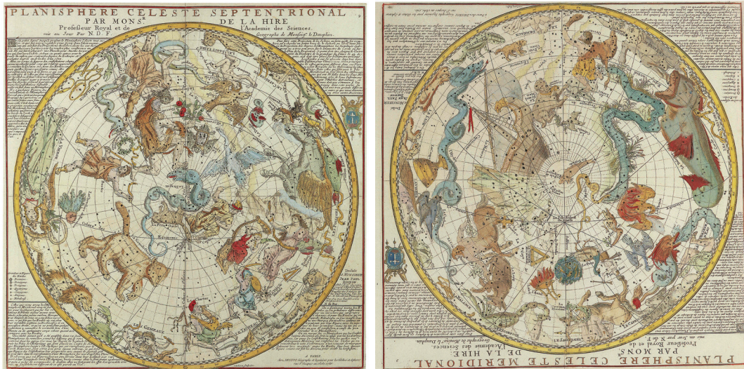
図 7: ド・ラ・イールによる天球図 (1705 年). 北天図 (1766 年の印刷), 南天図 (1760 年の印刷). どちらも 49.3 cm×61.6 cm. 正像であり, 中心は黄極, 赤道座標も点線で示されている. 千葉市立郷土博物館蔵. 画像は『星座の文化史』(千葉市立郷土博物館蔵, 1995) より.
