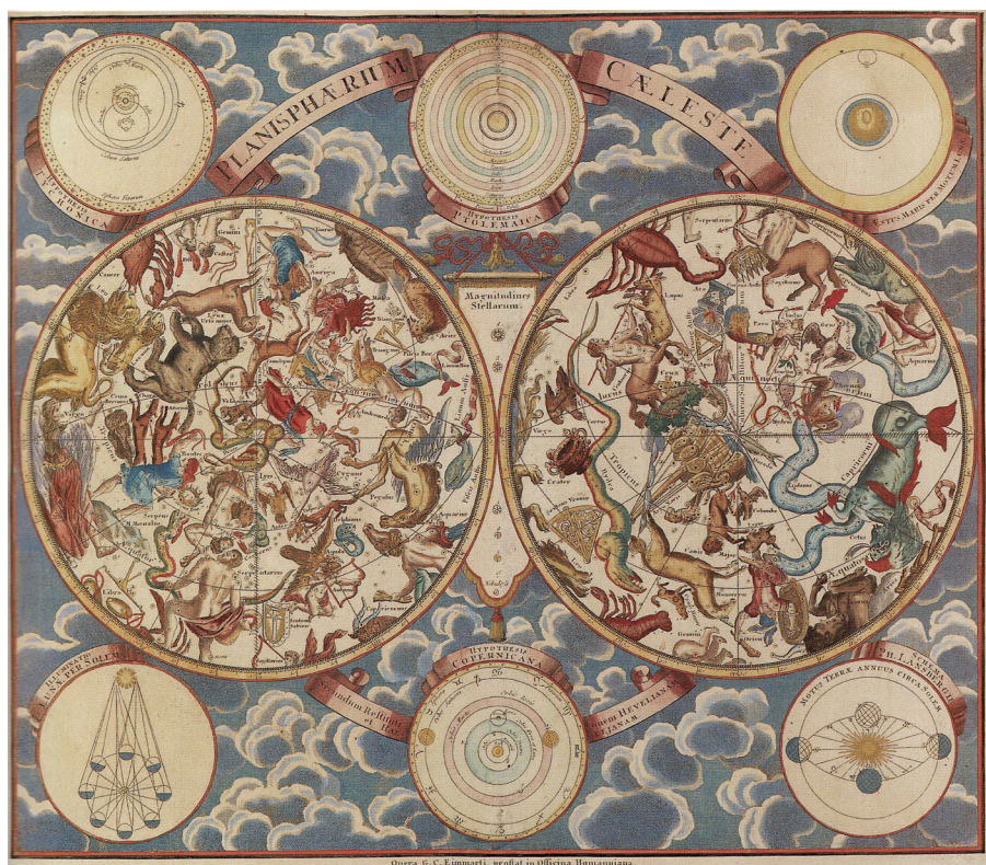
図 6: アインマルトによる天球図 (1705 年). 53.2 cm×64.4 cm. 反転星図, 黄道座標. 千葉市立郷土博物館蔵. 画像は『星座の文化史』(千葉市立郷土博物館蔵, 1995) より. Fig. 6: Celestial map by Georg Christoph Eimmart (1705).
