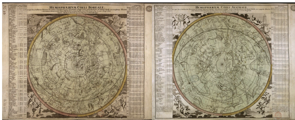
図 9: ドッペルマイヤーによる天球図 (1730 年). 正像であり, 赤道座標. 画像はインターネットから.
